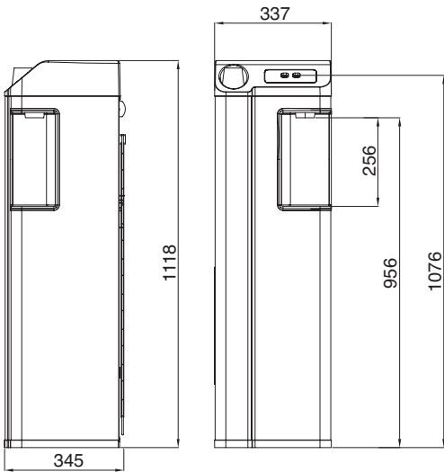
Dimensioni Dimensions Abmessungen Dimensions Dimensiones (mm)
