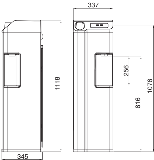
Dimensioni Dimensions Abmessungen Dimensions Dimensiones (mm)
